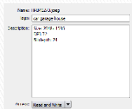
Plastique
