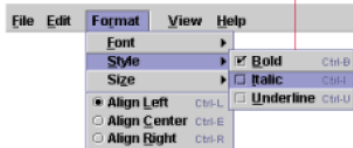
Submenu
