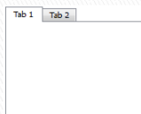
QTabWidget
